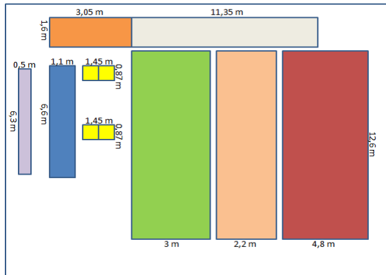
Gambar 6. Layout proses pengemasan tube sebelum ada usulan perancangan meja kerja
