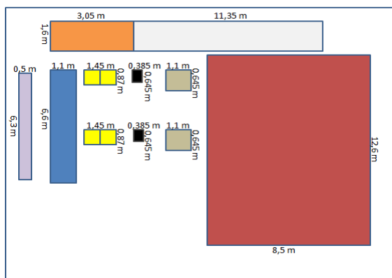
Gambar 7. Layout proses pengemasan tube setelah ada usulan perancangan meja kerja
